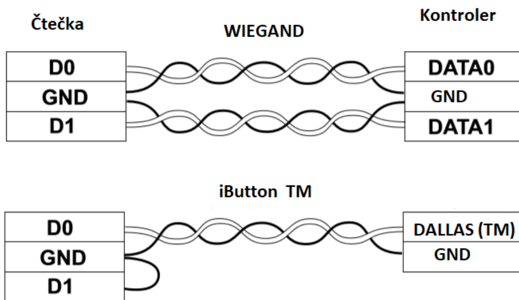
Obrázek č. 3: Přenosový protokol TM a WIEGAND 26.
