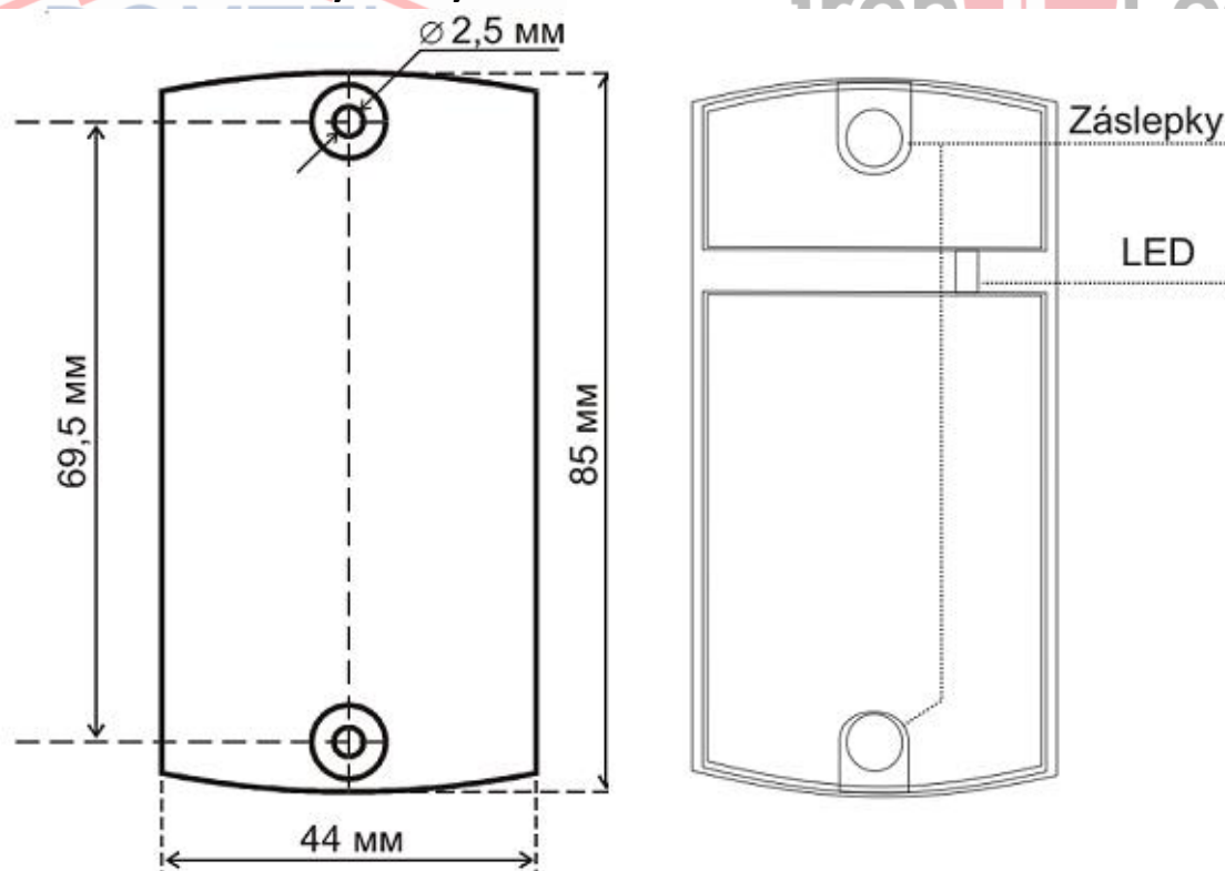
Obrázek č. 2: Rozměry čtečky MATRIX-II E
