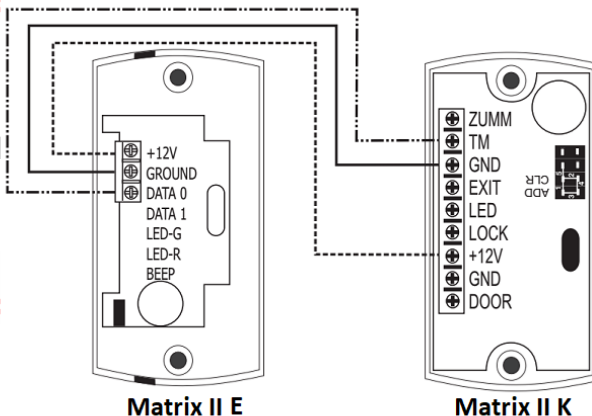
Obrázek č. 6: Propojení vodičů externí čtečka kontrolér.
