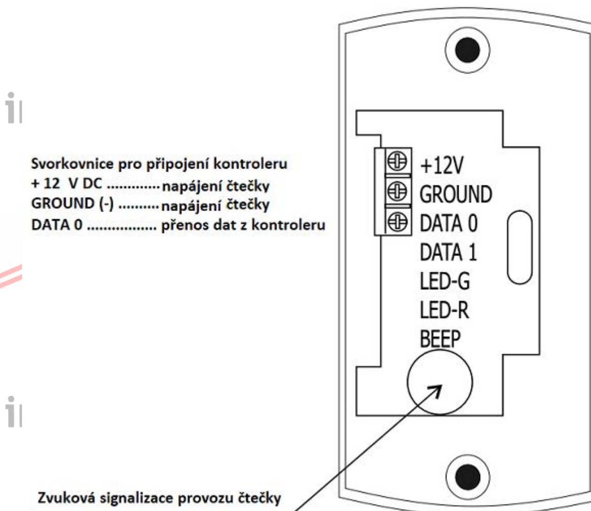
Obrázek č. 3: Svorkovnice čtečky MATRIX-II E.
