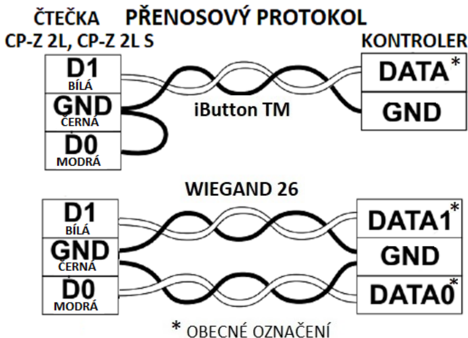
Obrázek č. 3: Zapojení vodičů čtečky.
