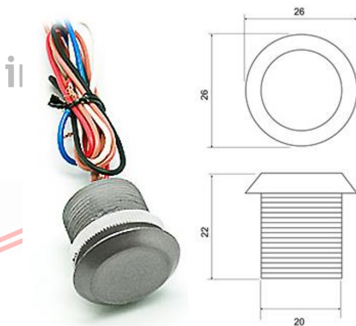
Obrázek č.1: Rozměry čtečky.
